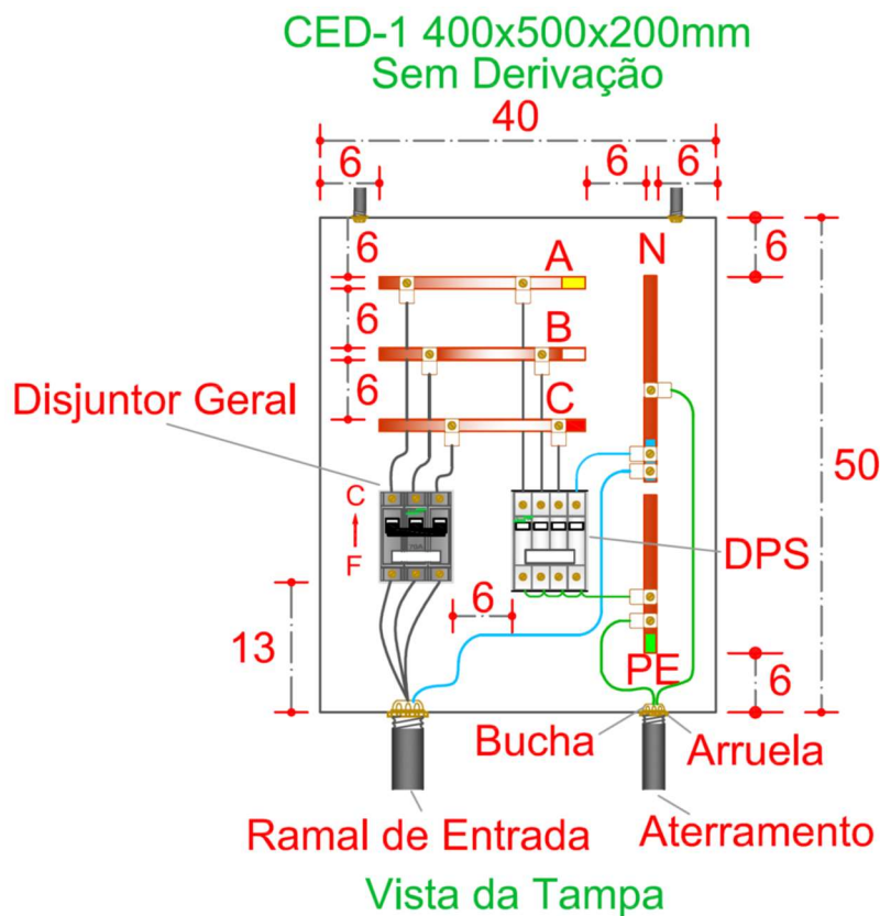
Figura 29(A) – Lay-out de CED-1 (400x500x200 mm) sem Derivação
