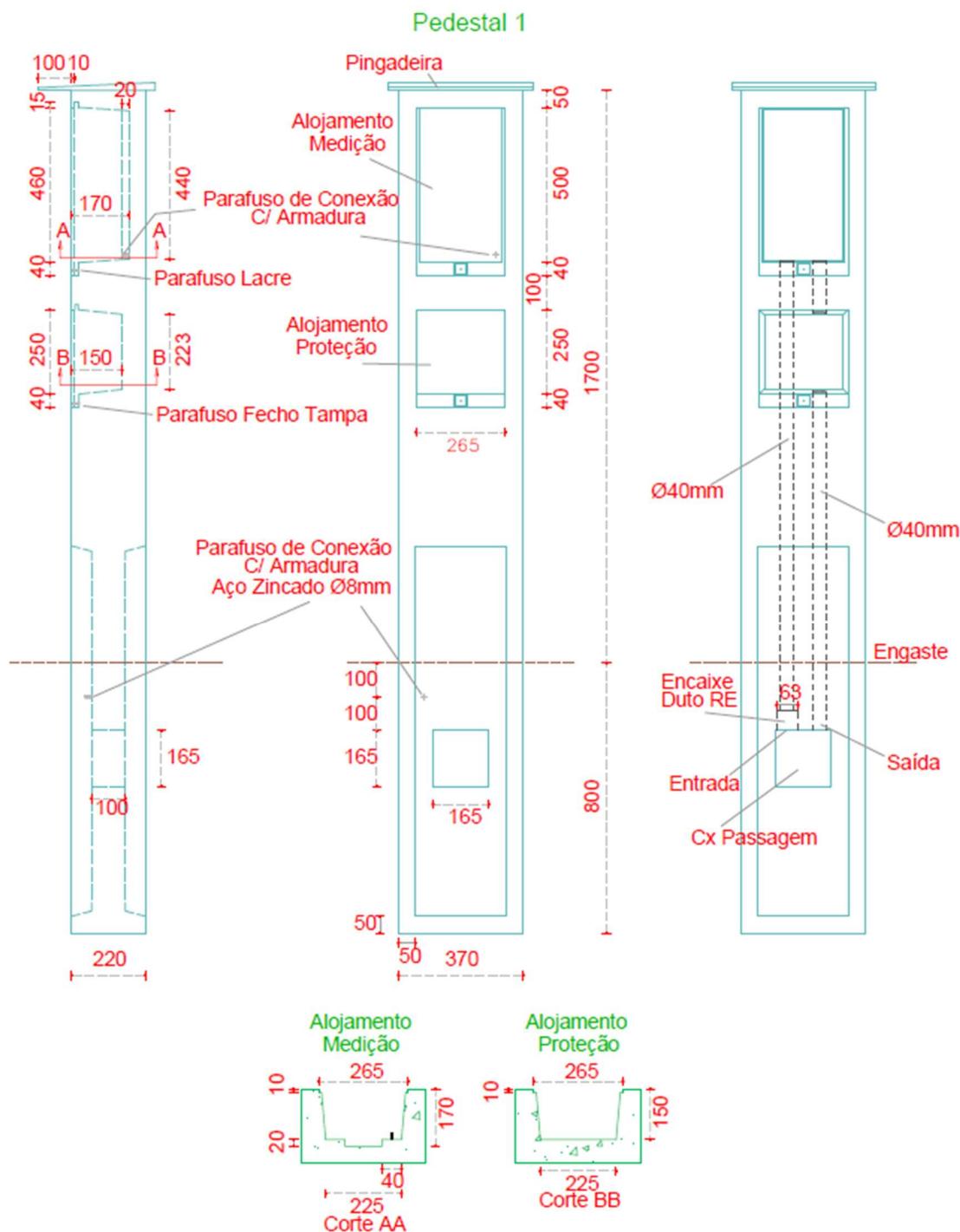
Figura 33(C) – Pedestal para Medição
