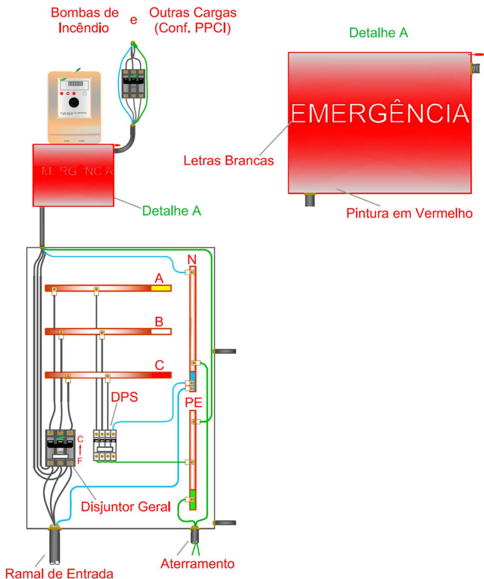
Figura 32 – Sistema de Emergência
